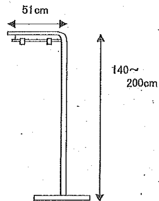
② サインスタンド(高)図
