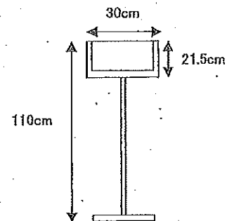
③ サインスタンド(低)図
